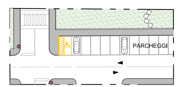
DETTAGLIO A INCROCIO TIPO CON SENSI DI MARCIA - STOP - PARK
