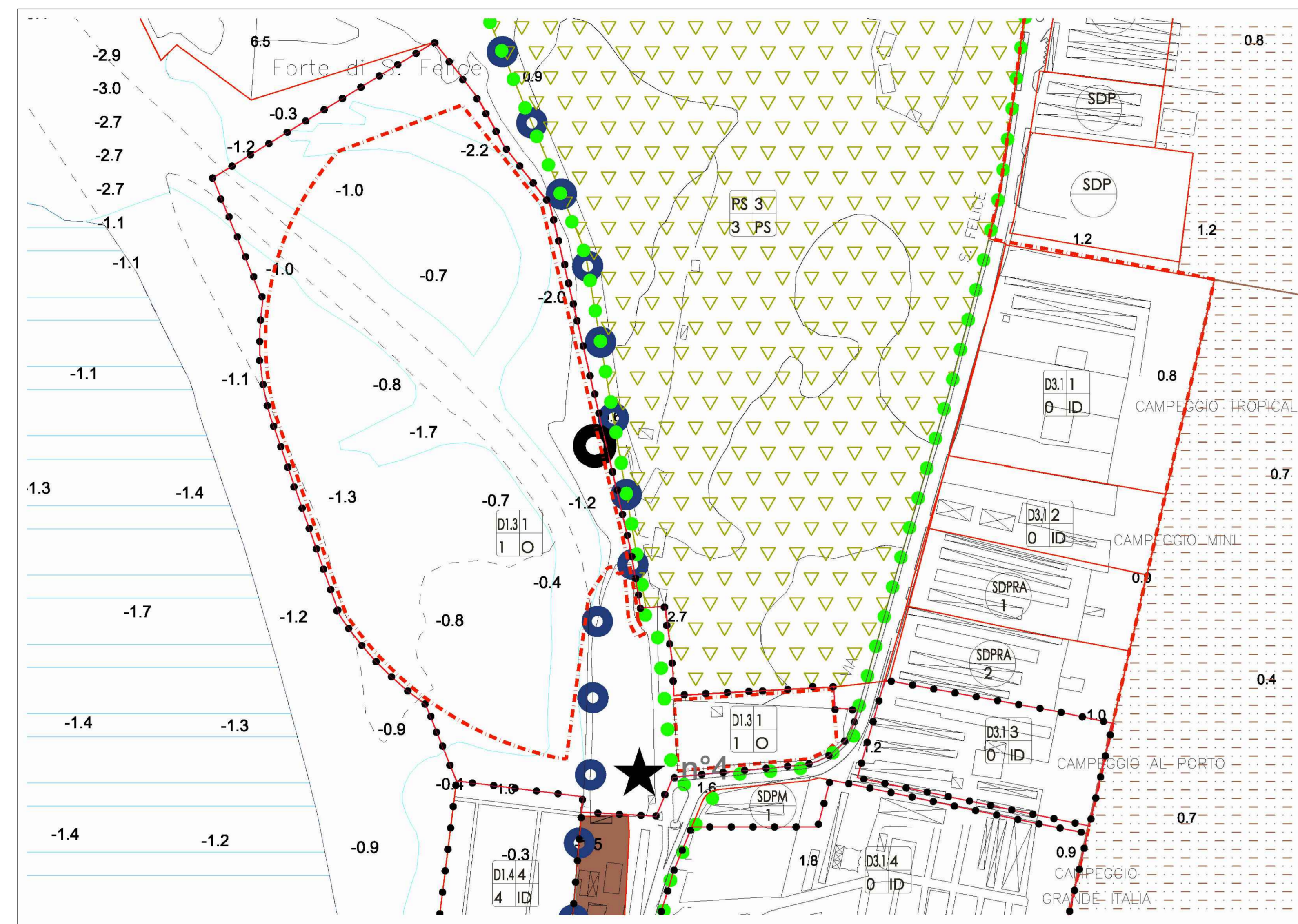
ESTRATTO P.R.G. TAV. 13.3.2 scala 1:2.000 (aggiornato con modifiche apportate dall'approvazione della Variante al P.R.G. Parco del Lungomare) (Approvato con D.G.R. n.3365 del 25 gennaio 2011)
